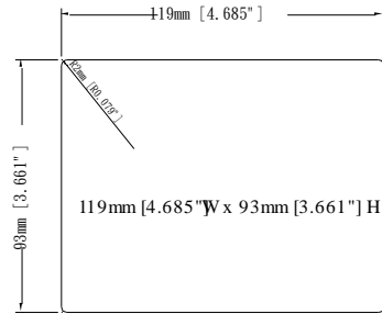
开孔尺寸图
