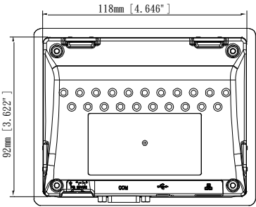
背视图
