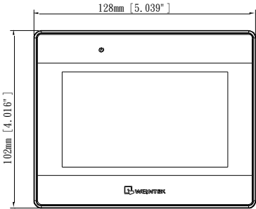
正视图
