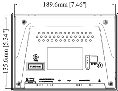
背视图
