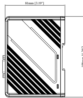
侧视图
