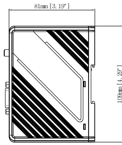
侧视图
