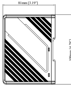
侧视图
