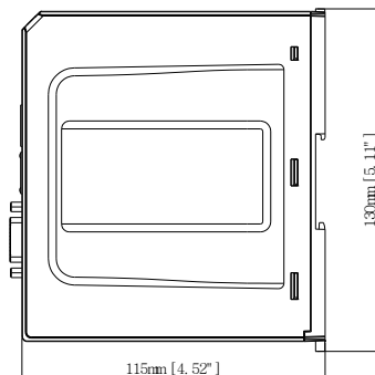
侧视图
