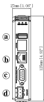
正视图
