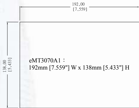
开孔尺寸图
