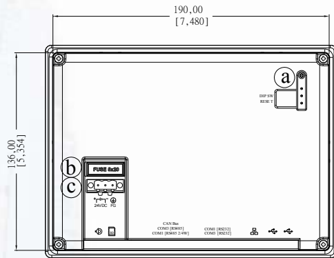
背视图
