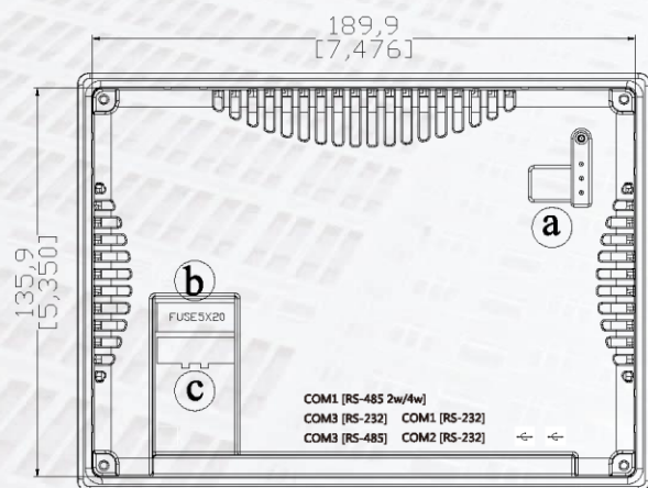
后视图
