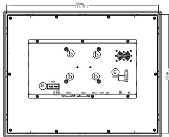
背视图
