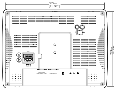
背视图
