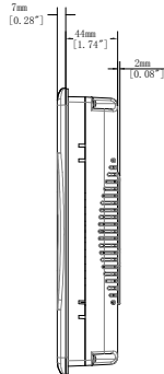
侧视图
